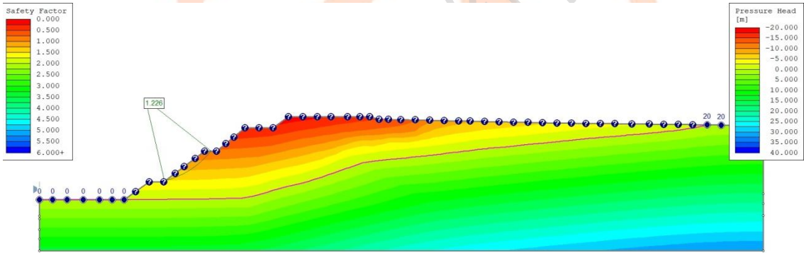
图 5-1 尾矿坝现状正常运行稳定计算
