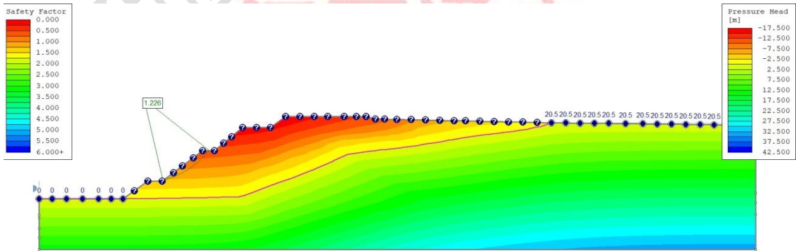
图 5-2 尾矿坝现状洪水运行稳定计算
