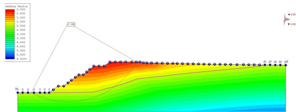
图 5-3 尾矿坝现状特殊运行稳定计算
