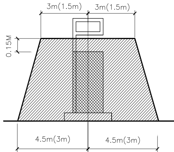
汽油加油机爆炸危险区域划分图
